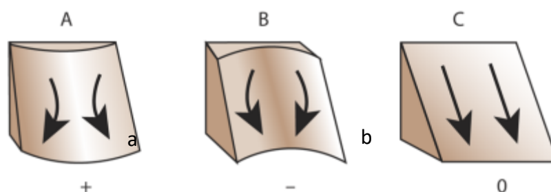
Figura 20. Curvatura horizontal: (a) Divergente; (b) Convergente; (c) Planar. Fonte: ESRI (2016).
