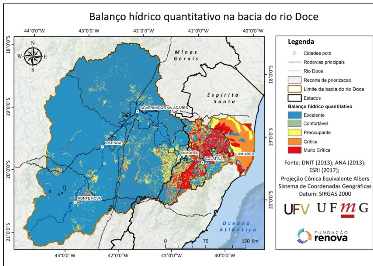
Figura 44. Balanço hídrico quantitativo na bacia do rio Doce.
