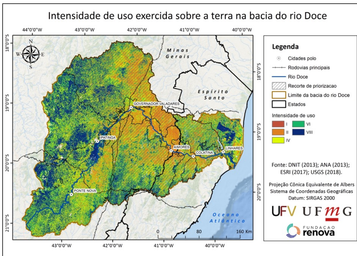
Figura 37. Intensidade de uso da terra na bacia do rio Doce.
