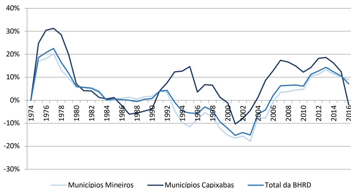
Figura 6. Evolução do rebanho bovino nos municípios mineiros e capixabas da bacia do rio Doce e total da bacia no período de 1974 a 2016.
