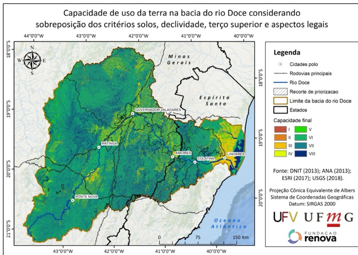
Figura 36. Capacidade de uso da terra na bacia do rio Doce considerando solos, declividade, terço superior e aspectos legais como fatores restritivos.
