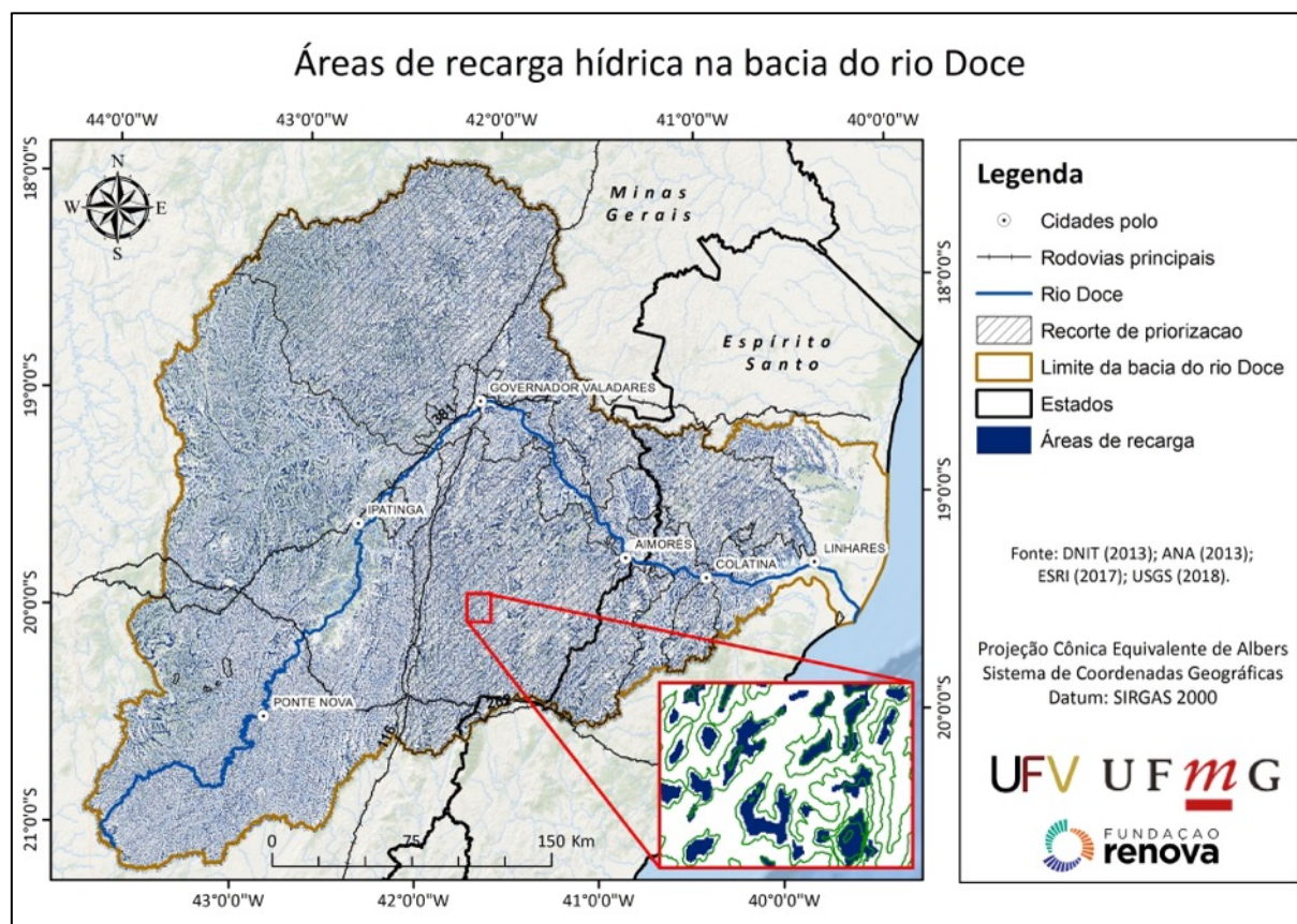
Figura 27. Áreas de recarga hídrica na bacia do rio Doce.
