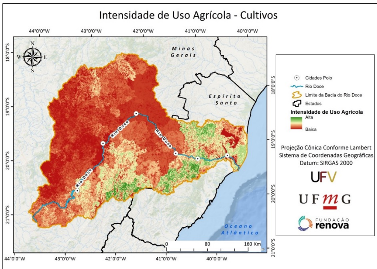
Figura 29. Intensidade histórica de uso agrícola (cultivos) para a bacia do Rio Doce considerando o ano de 1995.
