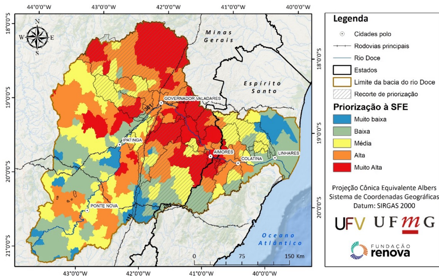
Figura 72. Mapa de áreas prioritárias para plantio total sem fins econômicos em escala municipal na bacia do rio Doce. Fonte: Elaborado pelas equipes UFV e UFMG.
