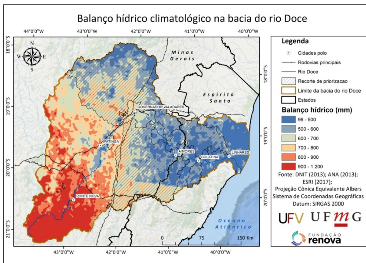
Figura 24. Balanço climatológico médio anual (TRMM e MODIS) para a bacia do rio Doce (2000 - 2014).
