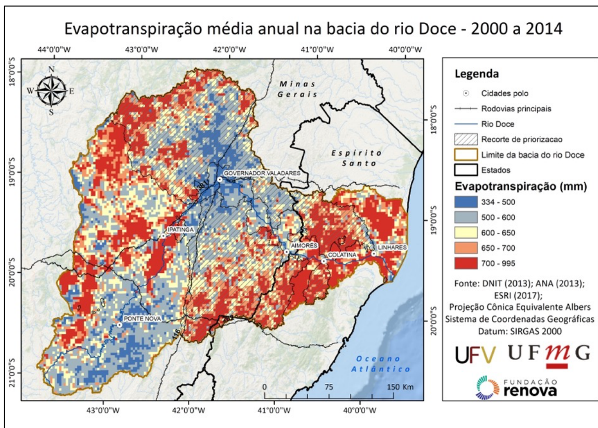
Figura 23. Evapotranspiração média anual (MODIS) para a bacia do rio Doce (2000 - 2014).
