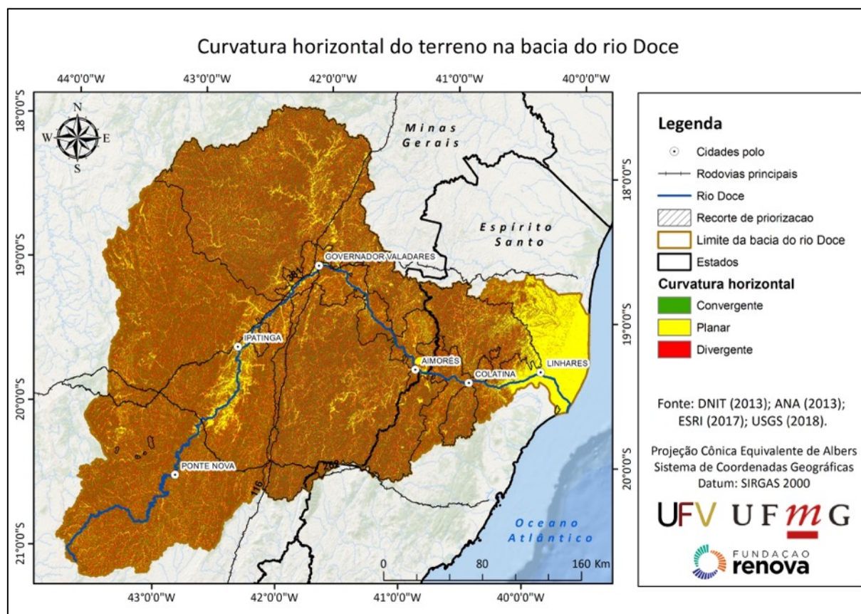
Figura 21. Curvatura horizontal do terreno na bacia do rio Doce.
