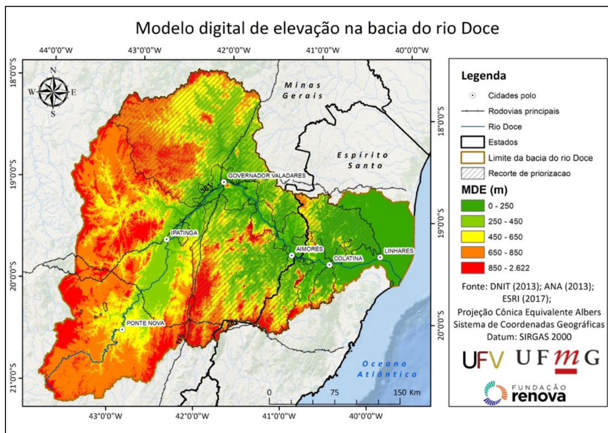
Figura 41. Modelo digital de elevação da bacia do rio Doce.
