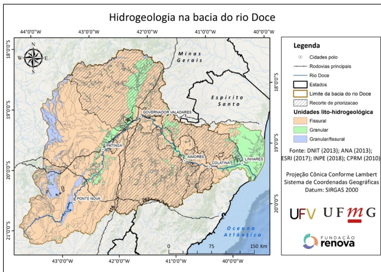
Figura 26. Unidades lito-hidrogeológicas da bacia do rio Doce.
